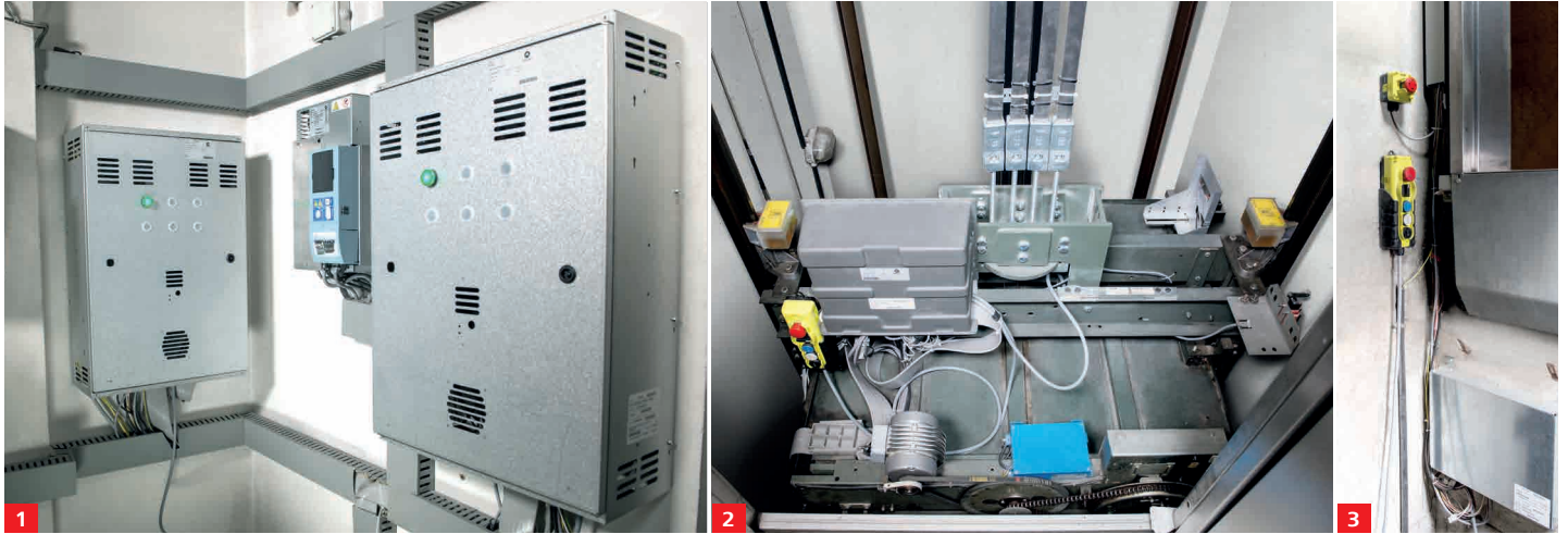
1: Aufbau im Maschinenraum | 2: Sicherheitselektronik auf dem Fahrkorbdach | 3: Sicherheitselektronik in der Schachtgrube
